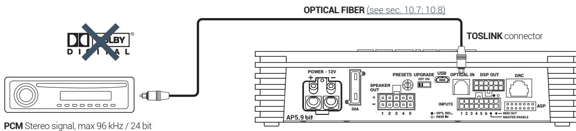
PCM Stereo signal, max 96 kHz / 24 bit
