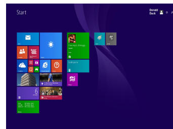
Windows 8/10
